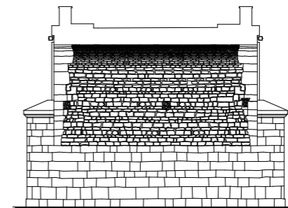
SEZIONE TRASVERSALE PARTICOLAREGGIATA
